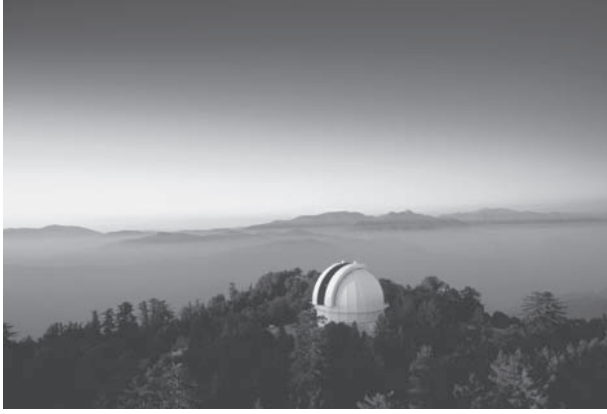
شكل ٢-١: قبة تليسكوب هوكر البالغ قطر مرآته ١٠٠ بوصة في مرصد ماونت ويلسون، والذي استخدمه إدوين هابل في قياس المسافات إلى المجرات.
